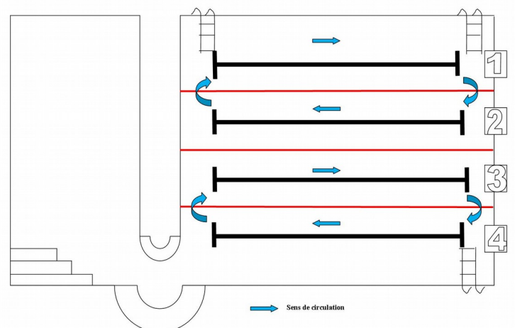
Plan d'utilisation du bassin pendant les créneaux nageurs
